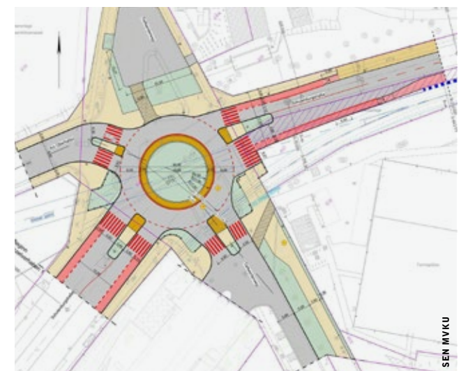
Abbildung 4, Kreisverkehr
