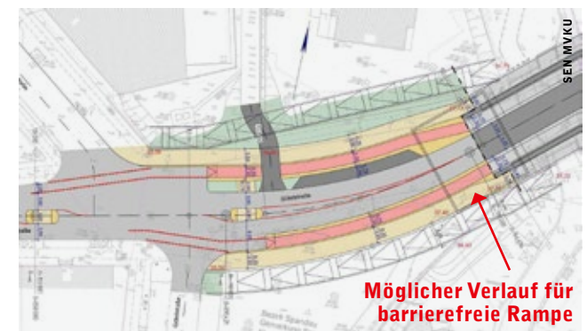
Abbildung 3, Barrierefreie Rampe
